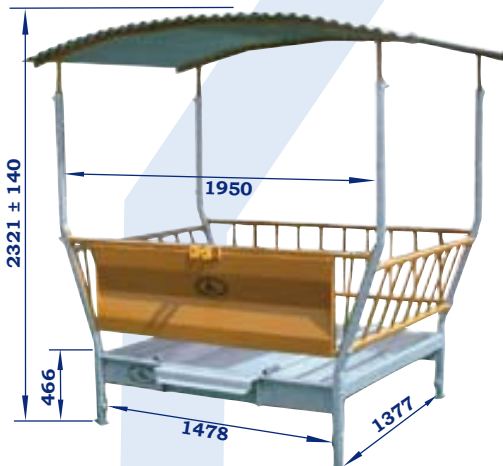
RMT 9801 Barrière arrière amovible
