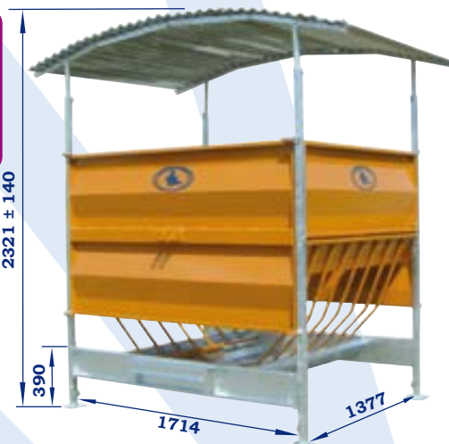
Grilles mobiles équipées de tôles pour protéger le dos des animaux des chutes de grains
